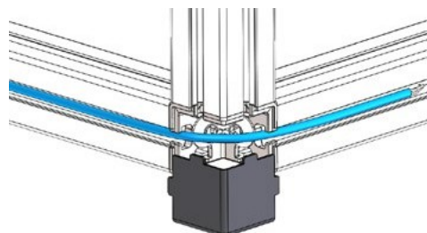
Rohový spoj FATH s 3D průchodem kabelů: spoj pro pravoúhlé trojrozměrné profilové konstrukce
